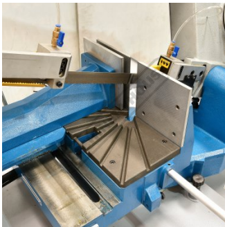
Dual Mitre Swivel Head
