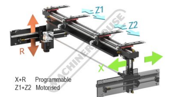
X R Programmable Z1 Z2 Motorised Backgauge
