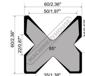
4V Die Block
