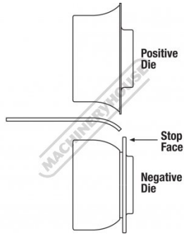
Die Drawing
