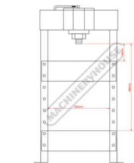
Dimensions
