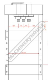
Dimensions
