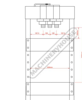
Dimensions
