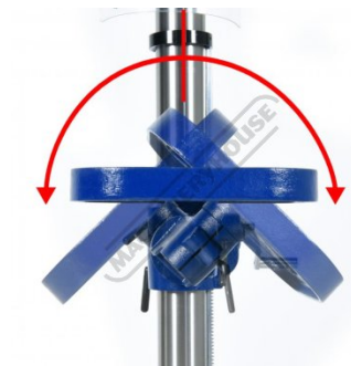
Tilting Table
