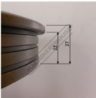
BE094 WHEEL OD 330 BORE 30.2
