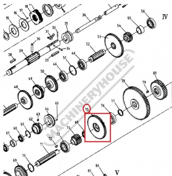
75 ..... C6266C-02716 ..... Gear ...
