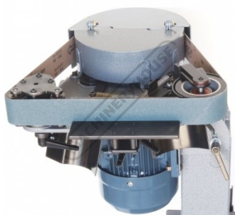
Optional Platen Table (L097)
